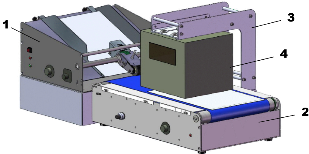
1- ALIMENTADOR 2- CINTA 3- SOPORTE UNIVERSAL 4- CABEZAL IMPRESOR
